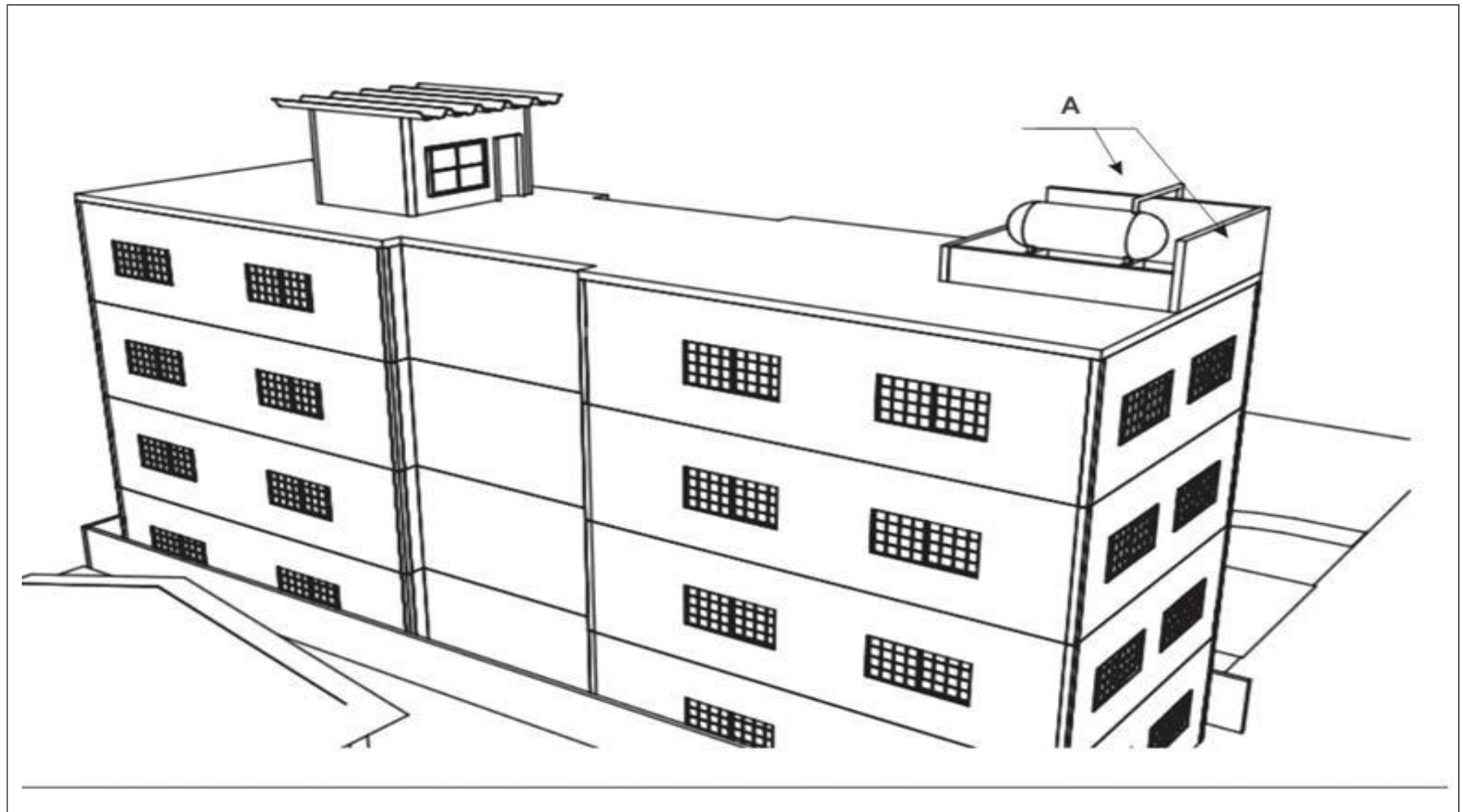
Figura 10b: Instalação de recipientes em teto e lajes de cobertura de edificações
