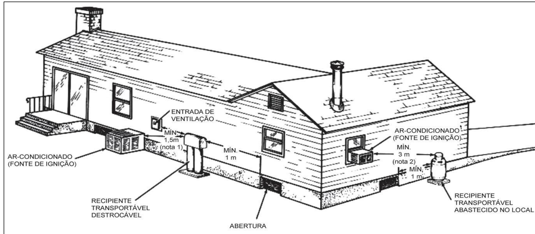
Figura 05: Instalação de recipientes transportáveis
