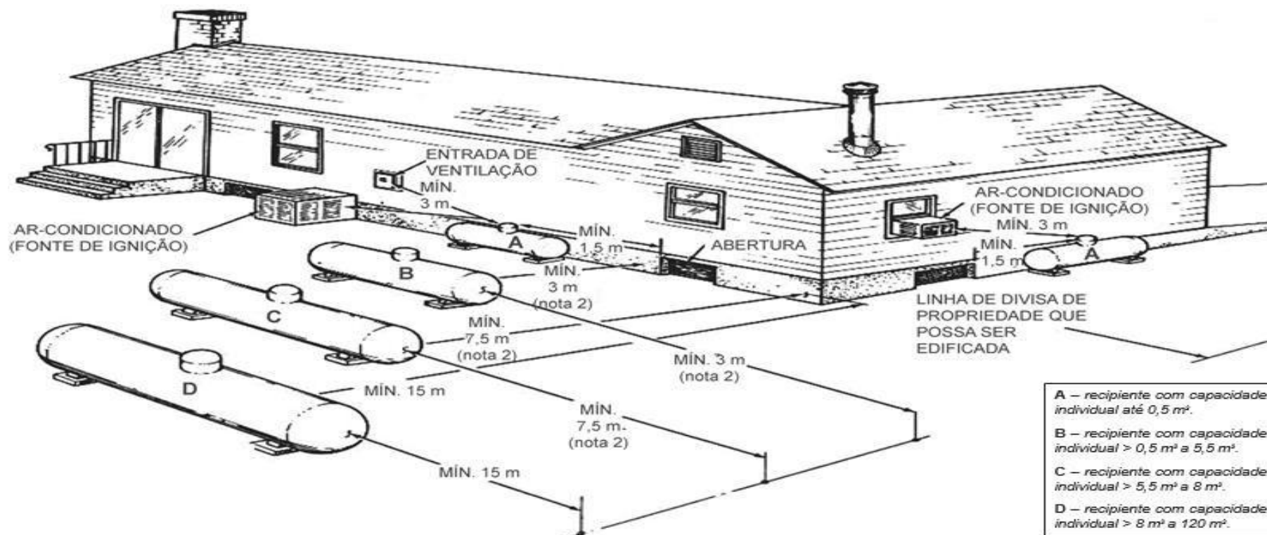
Figura 06: Instalação de recipientes estacionários de superfície
