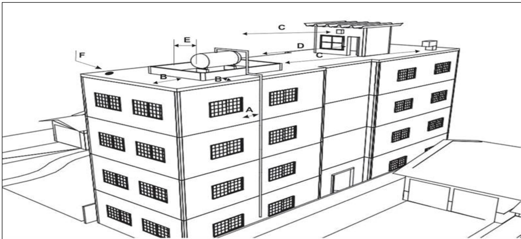
Figura 10a: Instalação de recipientes em teto e lajes de cobertura de edificações
